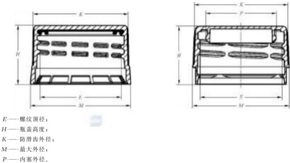
图 1 瓶盖尺寸示意图
